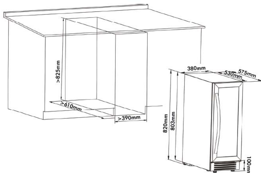
Instalação módulo único
