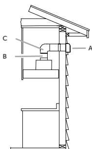
a) Tampa de ventilação para parede b) 8" (20,3 cm) duto redondo c) Joelho de 90°
