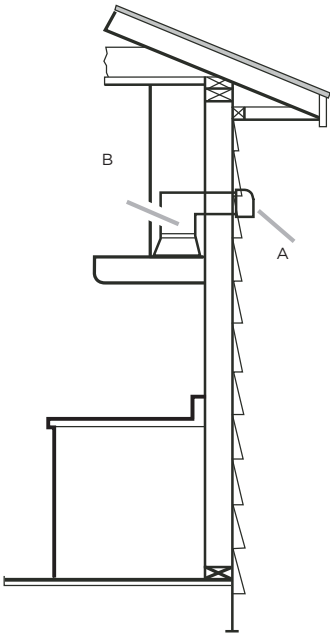
Saída de ar na parede (exaustão)
