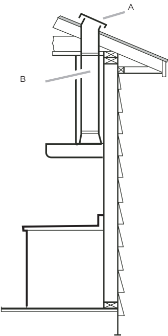
Saída de ar no teto (exaustão)
